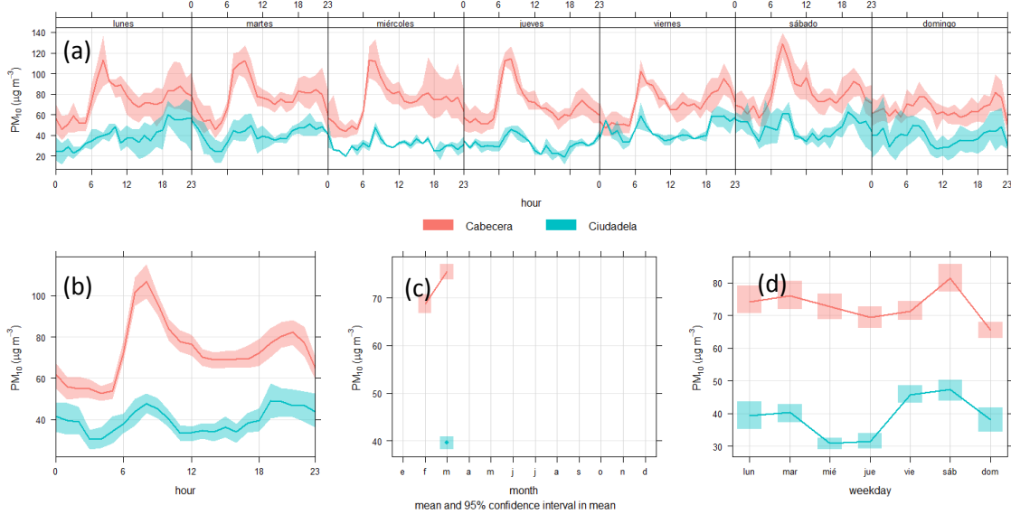
Figura 5 Comportamiento de PM10: (a) ciclo horario durante los diferentes días de la semana (b) comportamiento horario promedio, (c) promedio mensual y (d) comportamiento diario durante la semana. Nota: Para la estación Ciudadela solo se cuenta con datos para el periodo marzo 3 a marzo 21 por lo cual estos estadísticos pueden no ser representativos del comportamiento de la estación. Para la estación Cabecera se incluyeron datos desde el 25 de febrero para representar de mejor manera el comportamiento diario y horario del PM10.
