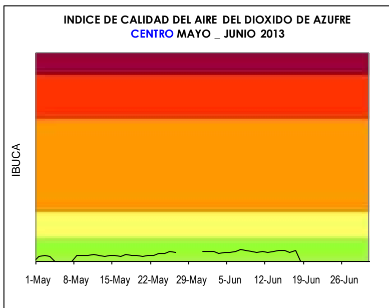
Fig8. Comportamiento SO 2 entre Mayo –Junio 2013
