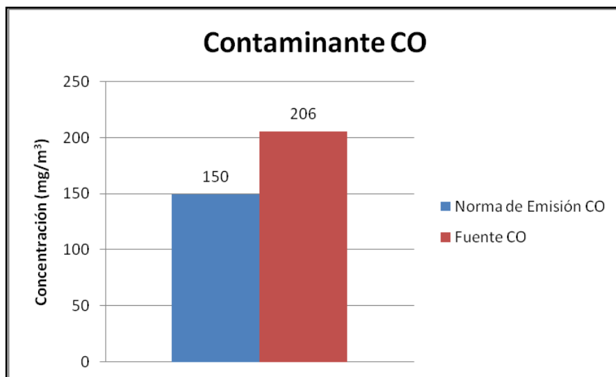
Gráfica 25. Concentración del contaminante CO en la empresa Sandesol
