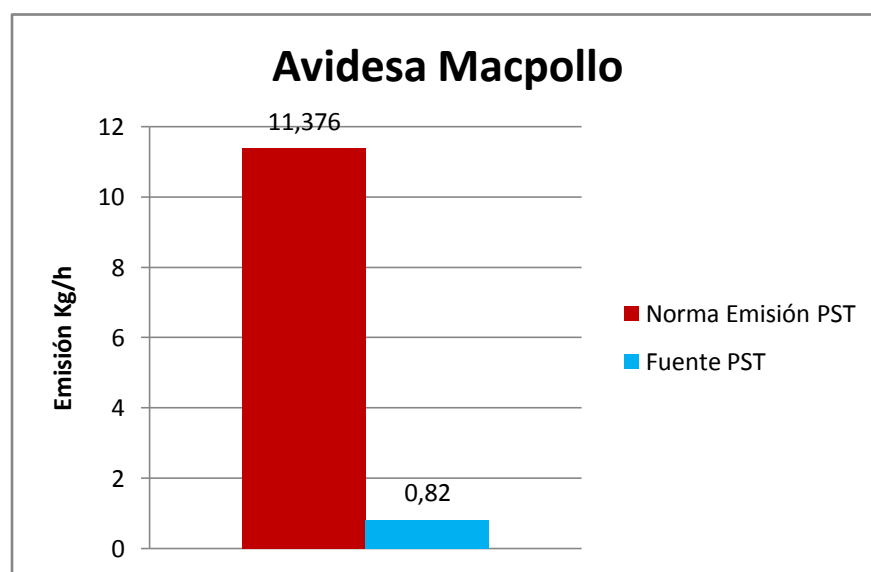
Gráfica 13. Comparación de la emisión de PST con los valores límites permisibles.
