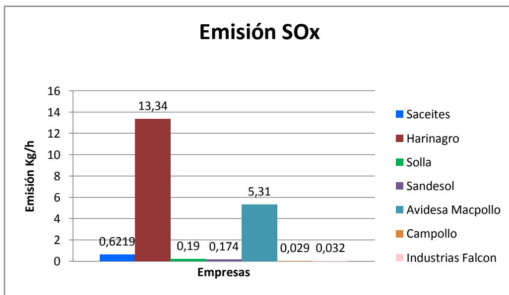
Gráfica 15. Emisión de SOx.
