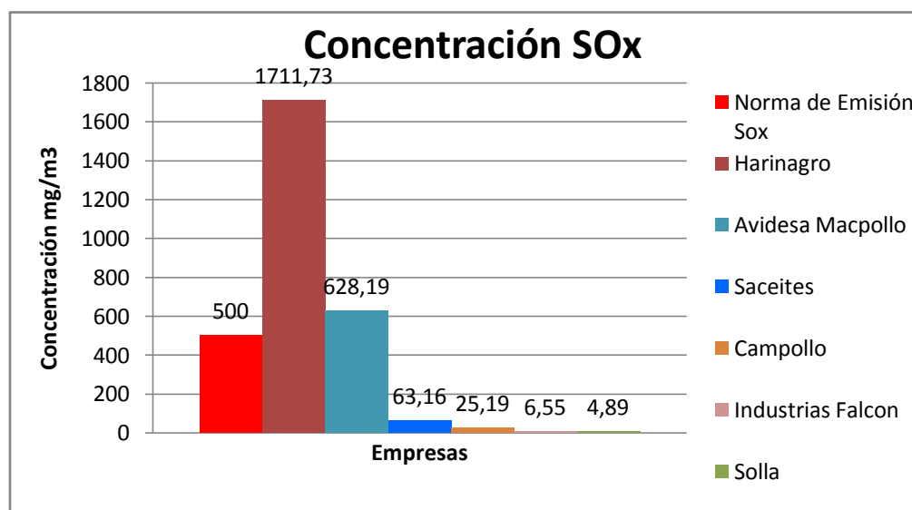
Gráfica 20. Concentración de SOx
