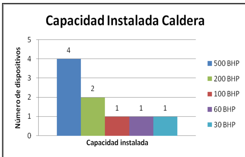
Gráfica 5. Capacidad Instalada de la Caldera
