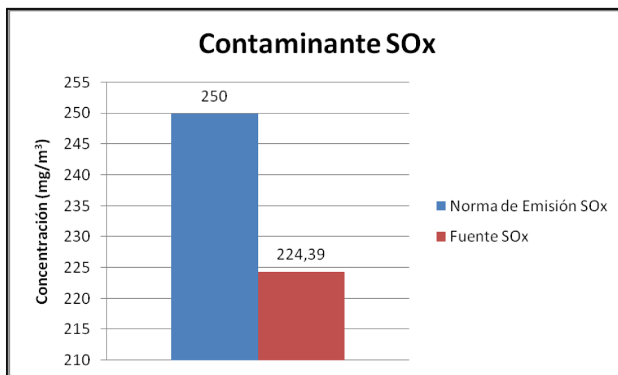
Gráfica 24. Concentración del contaminante SO x en la empresa Sandesol
