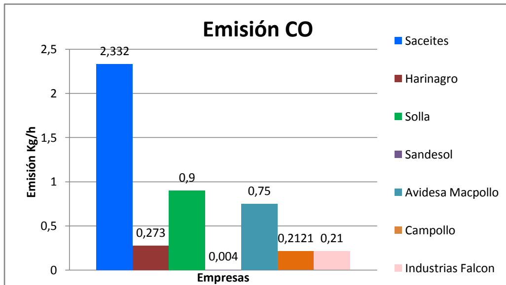
Gráfica 16. Emisión de CO.
