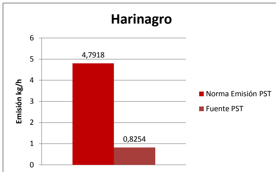
Gráfica 12. Comparación de la emisión de PST con los valores límites permisibles.
