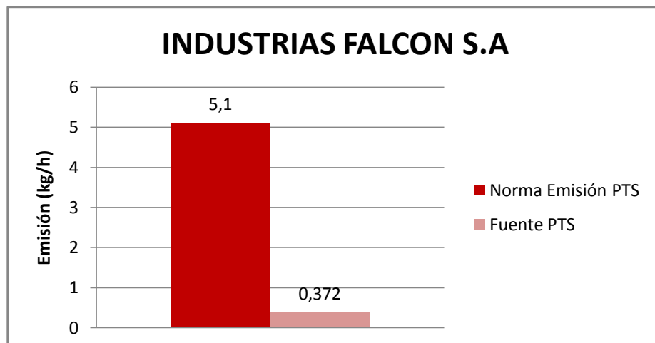
Gráfica 10. Comparación de la emisión de PST con los valores límites permisibles.
