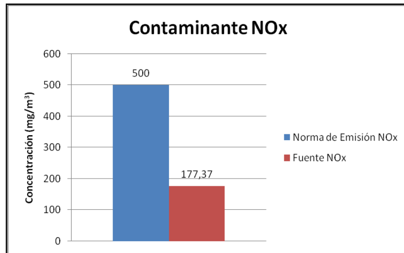
Gráfica 23. Concentración del contaminante NO x en la empresa Sandesol
