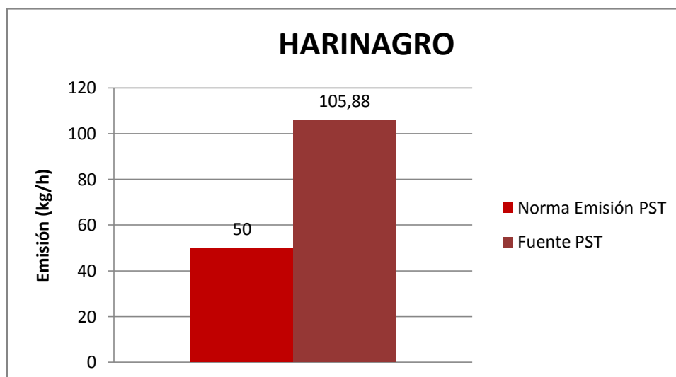
Gráfica 18. Concentración de PST
