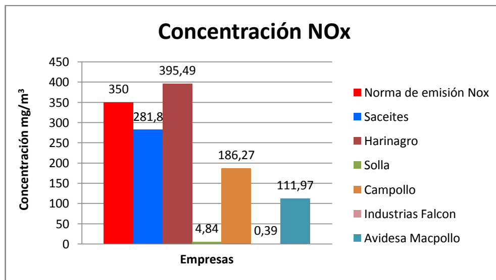
Gráfica 19. Concentración de NOx
