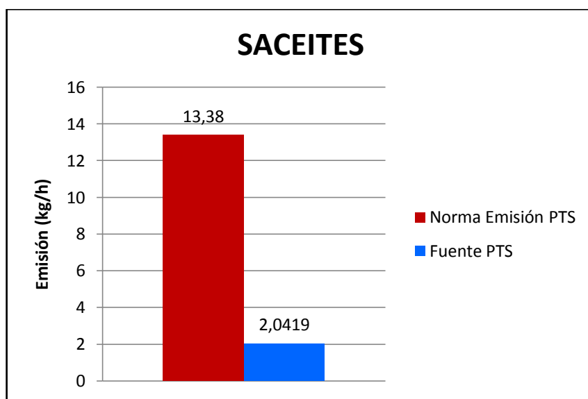
Gráfica 8. Comparación de la emisión de PST con los valores límites permisibles.
