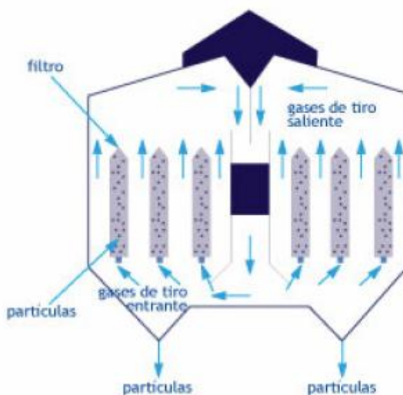
Figura 6. Diagrama de un Ciclón
