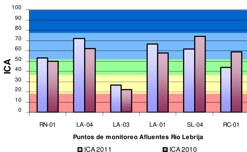
Grafica 23. Promedio Anual Índice de Calidad del Agua – Afluentes Río Lebrija
