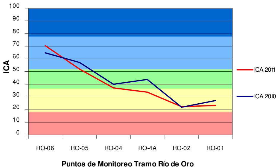
Grafica 9. Promedio Anual Índice de Calidad del Agua - Río de Oro
