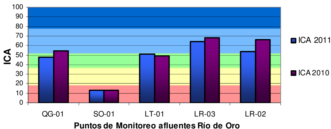
Grafica 11. Promedio Anual Índice de Calidad del Agua - Afluentes parte Alta y Media Río de Oro
