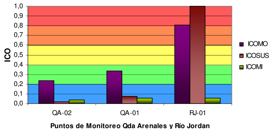
Grafica 28. Promedio Índices de Contaminación del Agua 2011 - Qda Arenales y Río Jordán
