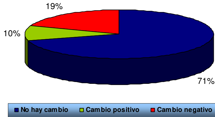
Grafica 2. Porcentaje de calidades anuales ICA 2011-2010
