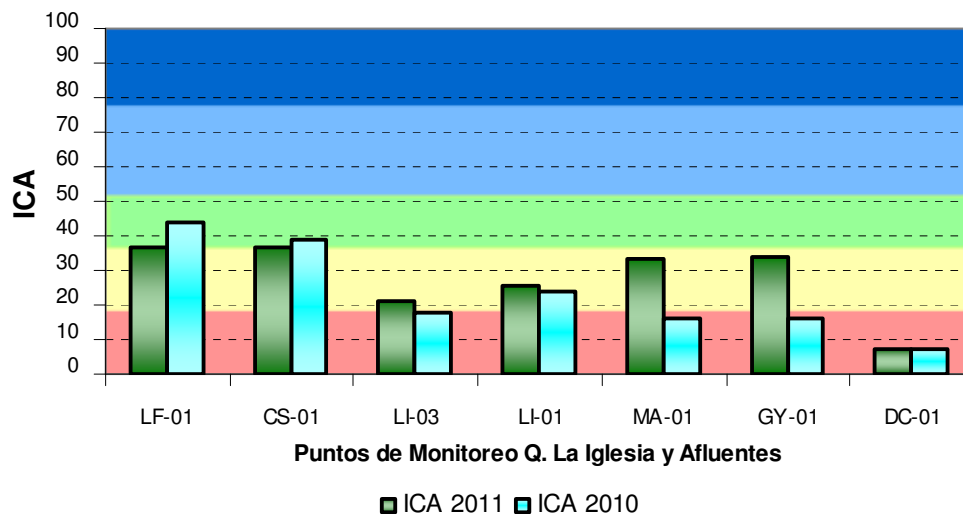
Gráfica 17. Promedio Anual Índice de Calidad del Agua – Quebrada La Iglesia y sus afluentes
