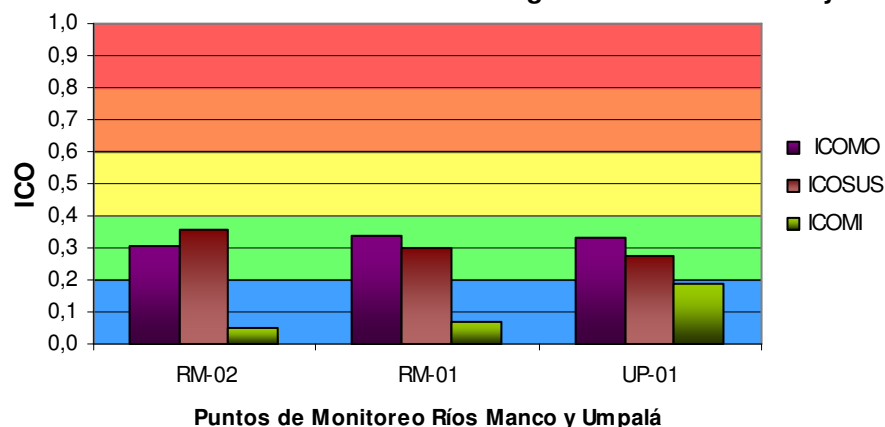
Grafica 26. Promedio Índices de Contaminación del Agua 2011 - Ríos Manco y Umpalá
