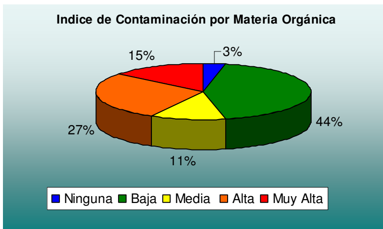
Grafica 4. Promedio Índice de Contaminación por Sólidos Suspendidos
