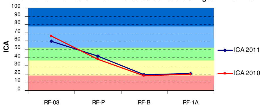
Grafica 13. Promedio Anual Índice de Calidad del Agua – Río Frío
