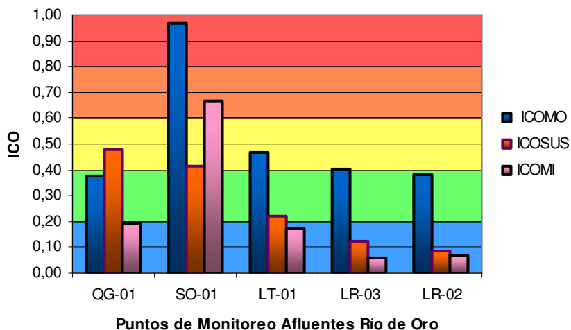
Grafica 12. Promedio Índices de Contaminación del Agua 2011- Afluentes Río de Oro
