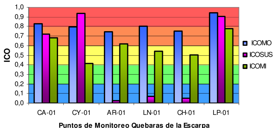
Grafica 20. Promedio Índices de Contaminación del Agua 2011- Quebradas de la escarpa
