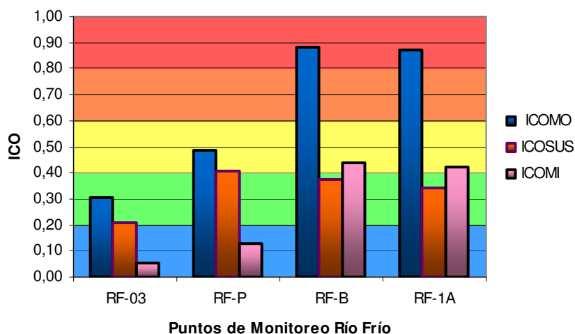
Grafica 14. Promedio Índices de Contaminación del Agua 2011- Río Frío
