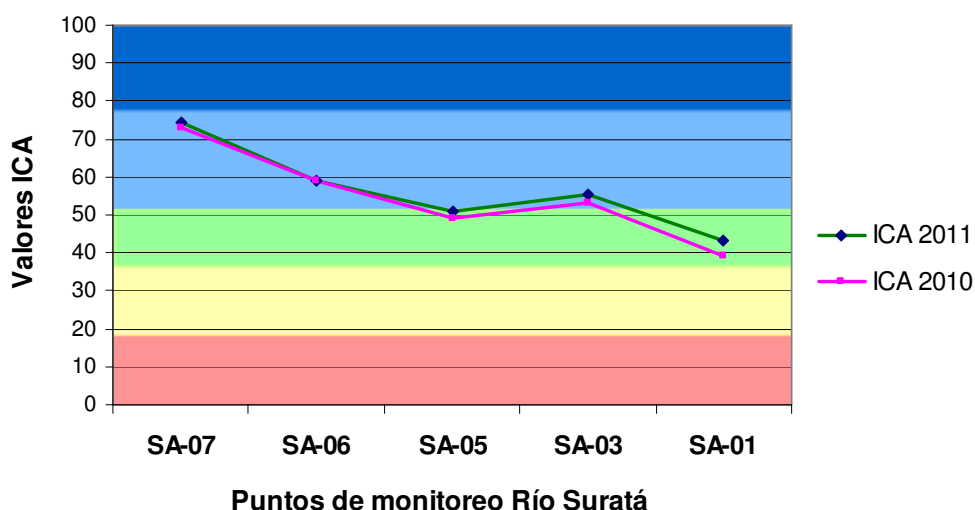
Grafica 7. Promedio Anual Índice de Calidad del Agua - Río Suratá
