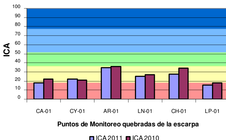
Corporación Autónoma Regional para la Defensa de la Meseta de Bucaramanga Grafica 19. Promedio Anual Índice de Calidad del Agua – Quebradas de la escarpa
