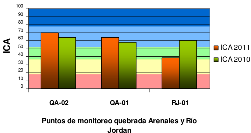
Grafica 27. Promedio Anual Índice de Calidad del Agua – Qda Arenales y Río Jordán
