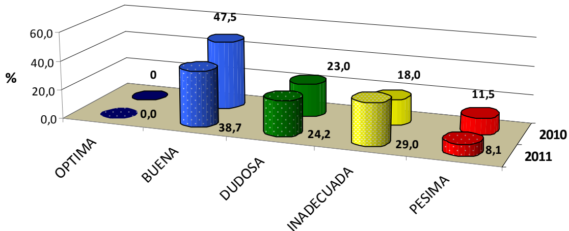
Grafica 2. Porcentaje de calidades anuales ICA 2011-2010
