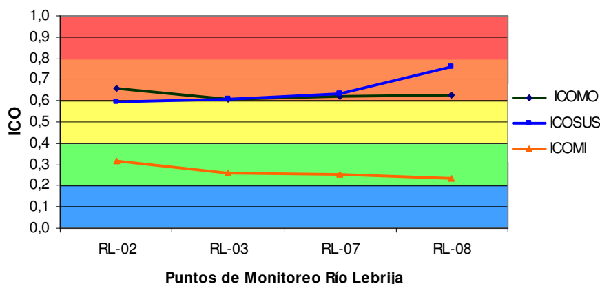
Corporación Autónoma Regional para la Defensa de la Meseta de Bucaramanga Grafica 22. Promedio Índices de Contaminación del Agua 2011- Río Lebrija
