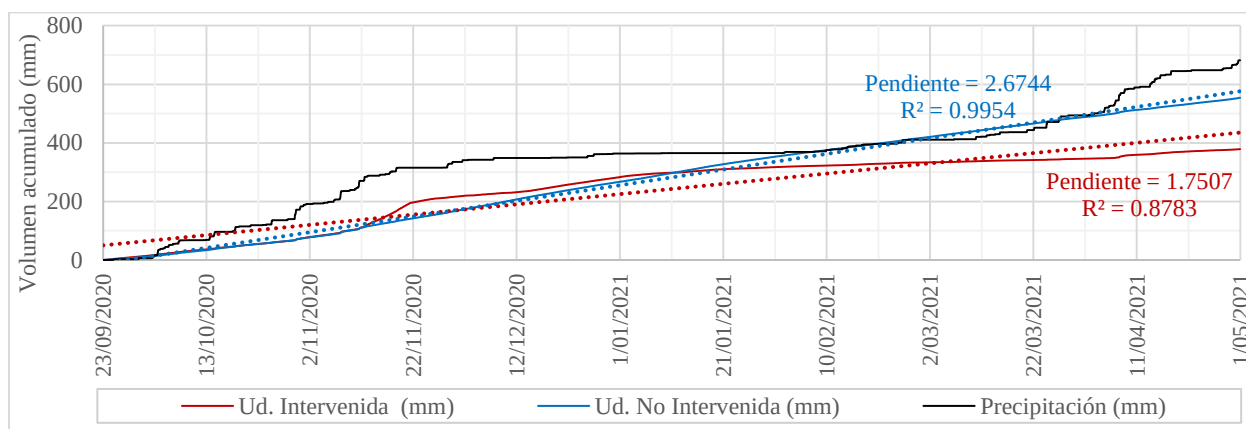
Figura 59. Curvas acumuladas de precipitación y descarga para el cuarto período continuo de registros (desde septiembre de 2020 hasta abril de 2021).
