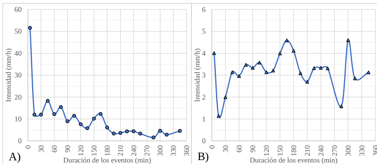
Figura 36. Curvas de intensidad y duración de las lluvias registradas. A) Máxima. B) Promedio.
