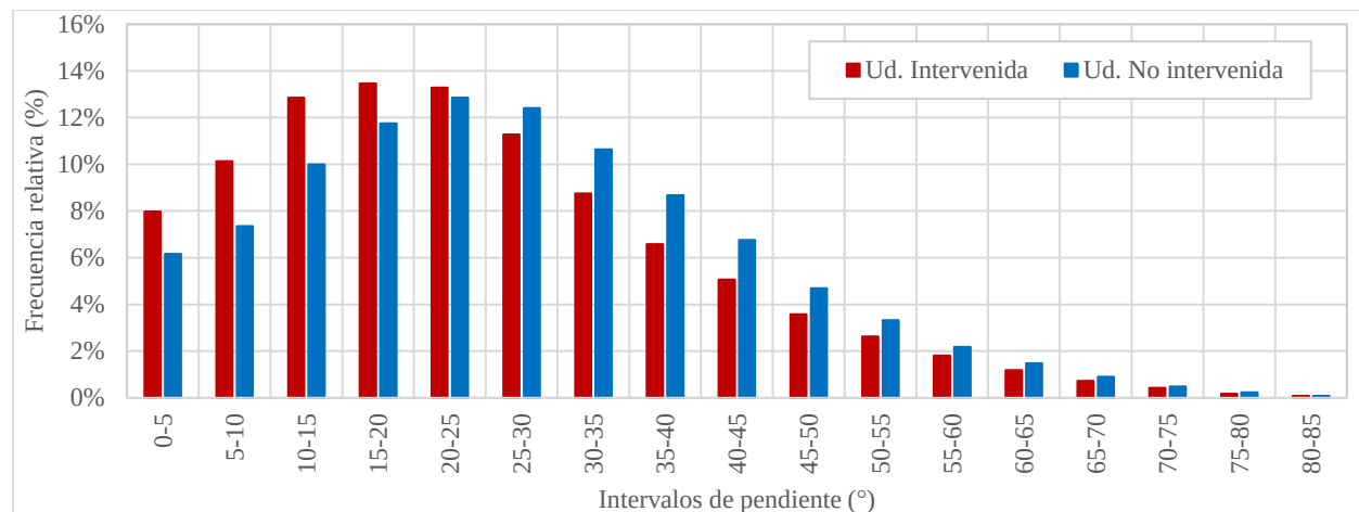
Figura 26. Histogramas de valores de pendiente de las unidades.
