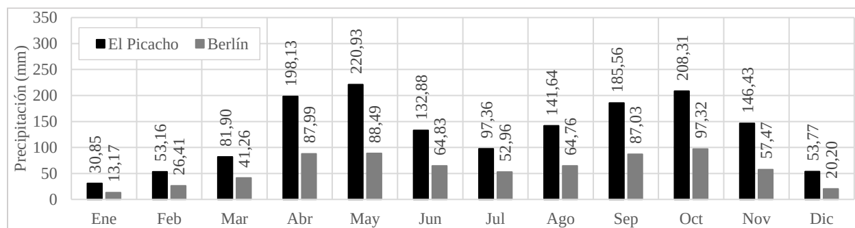
Figura 32. Régimen promedio anual de la precipitación en la zona de estudio.
