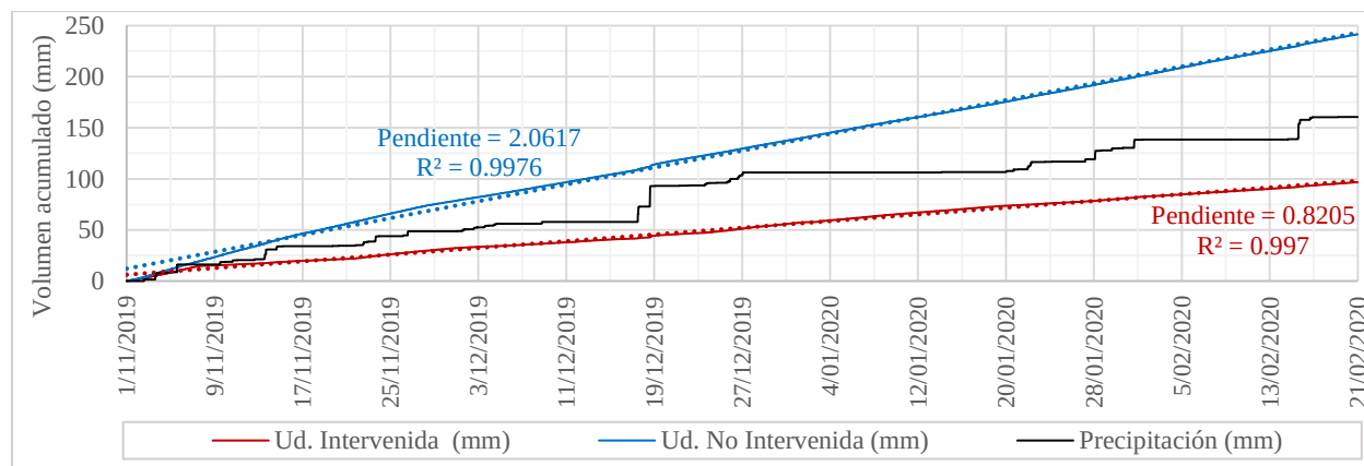
Figura 56. Curvas acumuladas de precipitación y descarga para el primer período continuo de registros (desde noviembre de 2019 hasta febrero de 2020).
