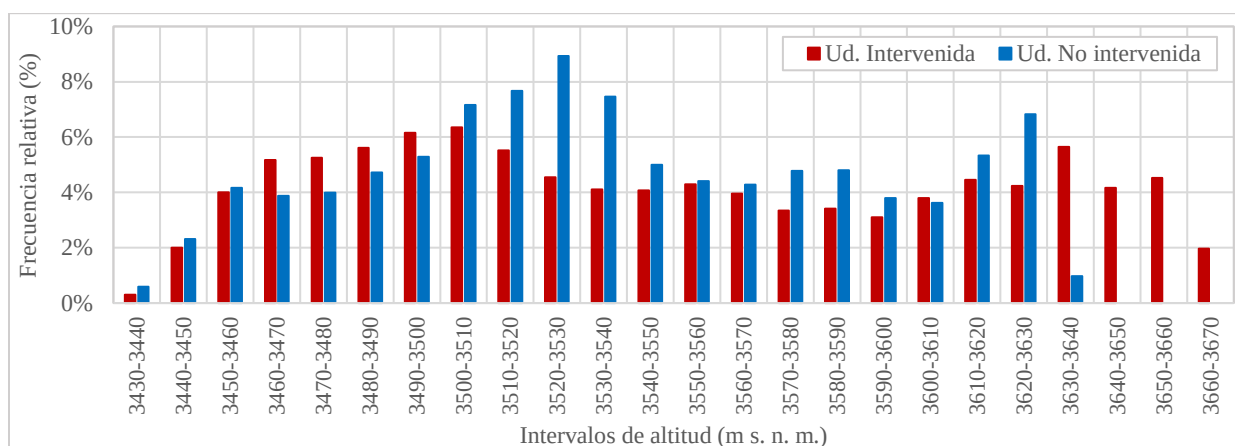
Figura 23. Histogramas de valores de altimetría de las unidades.
