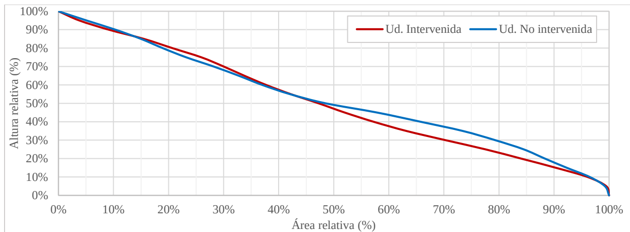
Figura 24. Curvas hipsométricas.
